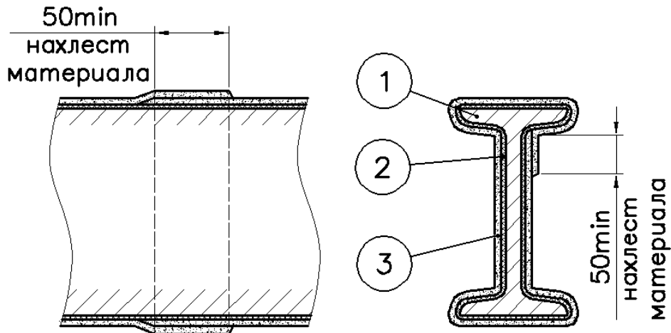
Рис. 1. Устройство покрытия на поверхности металлоконструкций.
